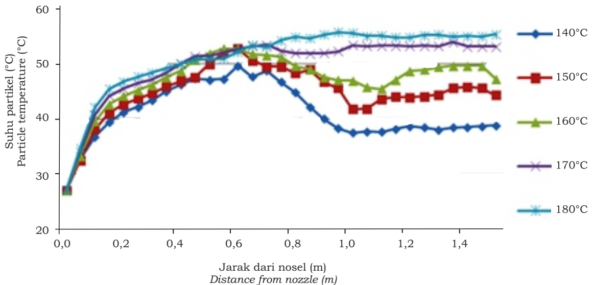
Gambar 9. Prediksi profil suhu partikel tepung lateks pada berbagai suhu udara pengering dan kadar air lateks
