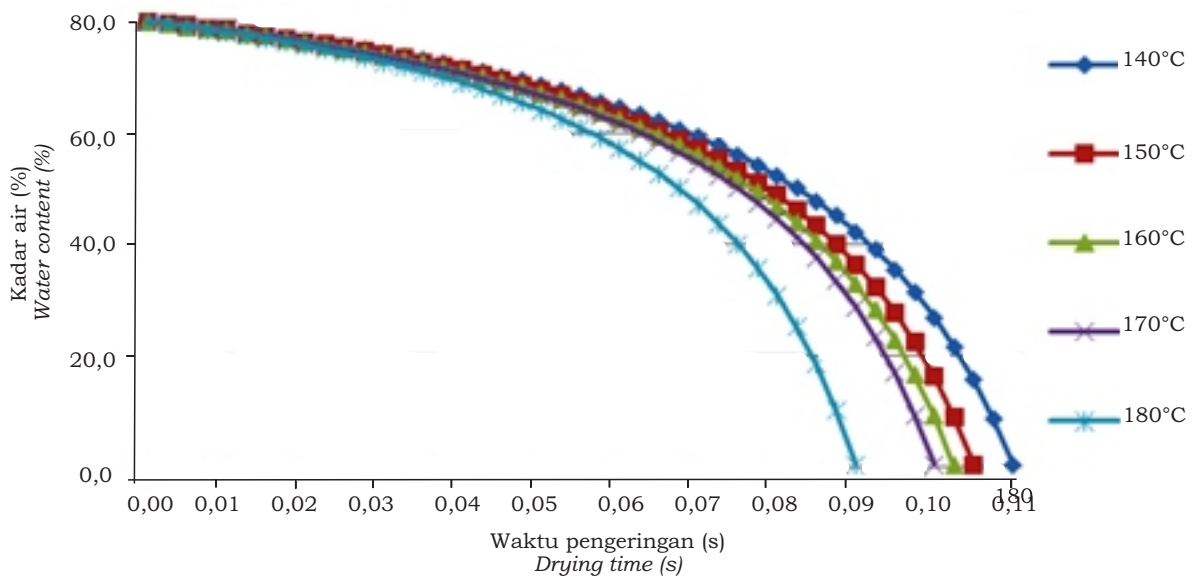
Gambar 6. Profil kadar air tetesan lateks pada berbagai suhu udara pengering dan kadar air lateks
