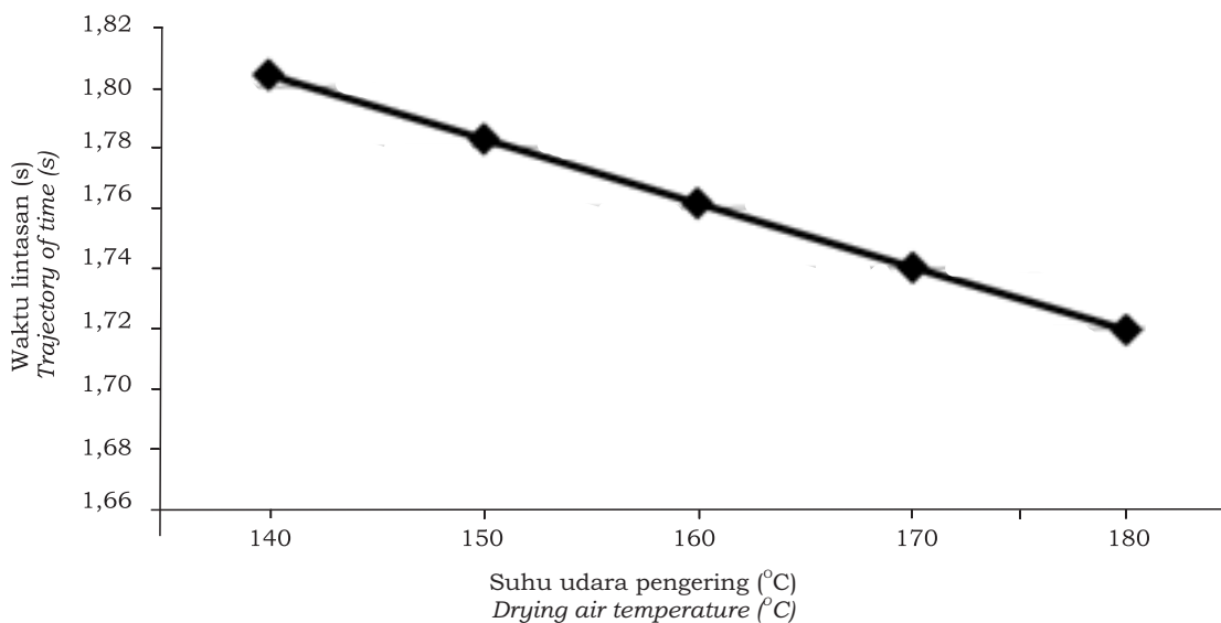
Gambar 7. Waktu lintasan lateks di ruang pengering berbentuk silinder
