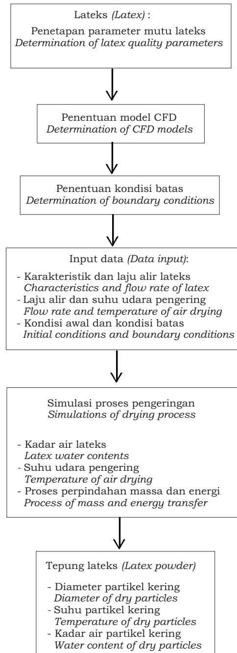
Gambar 1. Diagram alir simulasi pengeringan lateks
