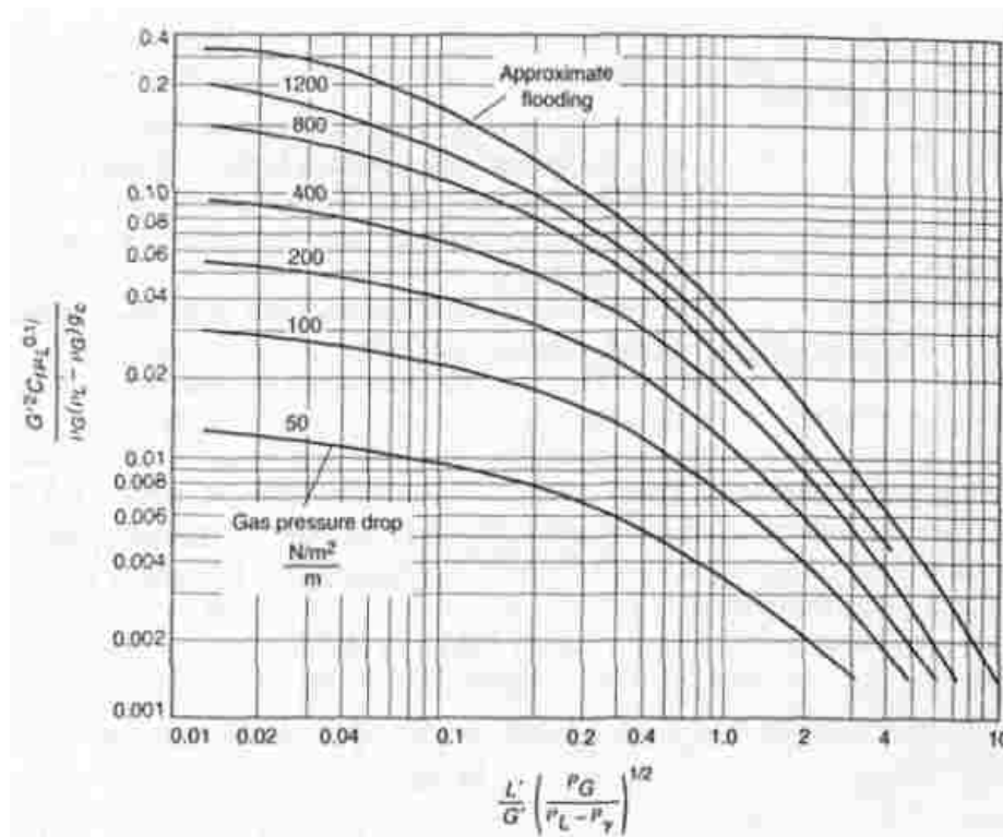
Gambar 2. Grafik untuk perhitungan nilai G' Figure 2. Graphic for calculating G'
